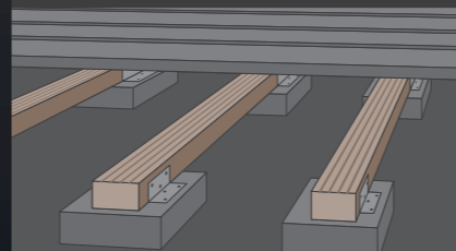
Unterkonstruktion Substructure
